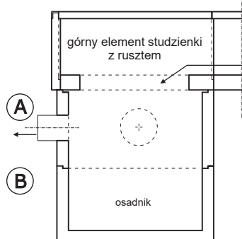
rys. 2 studzienka osadnikowo-odpływowa
