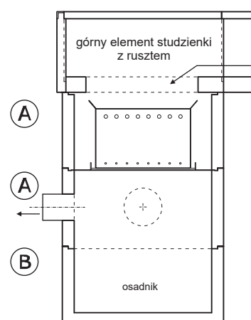
rys. 4 studzienka osadnikowo-odpływowa
