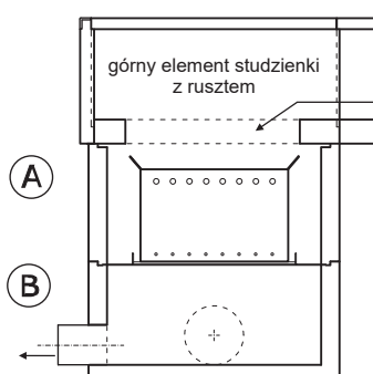
rys. 3 studzienka odpływowa
